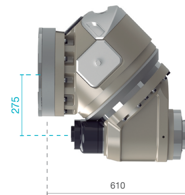
Cabezal 45° 45° head
